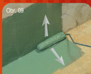
Obr. 09 Nanášení - aplikace / Nanášenie - aplikácia 25 Nanést první vrstvu Tekuté lepenky. Naniesť prvú vrstvu Tekutej lepenky.
